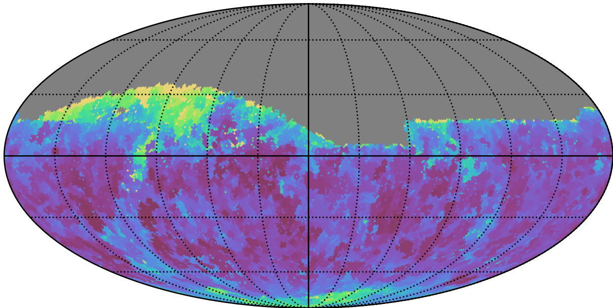
weather_cloudso36v3.4_10yrs Yr 1 z band: Min seeingGeom
