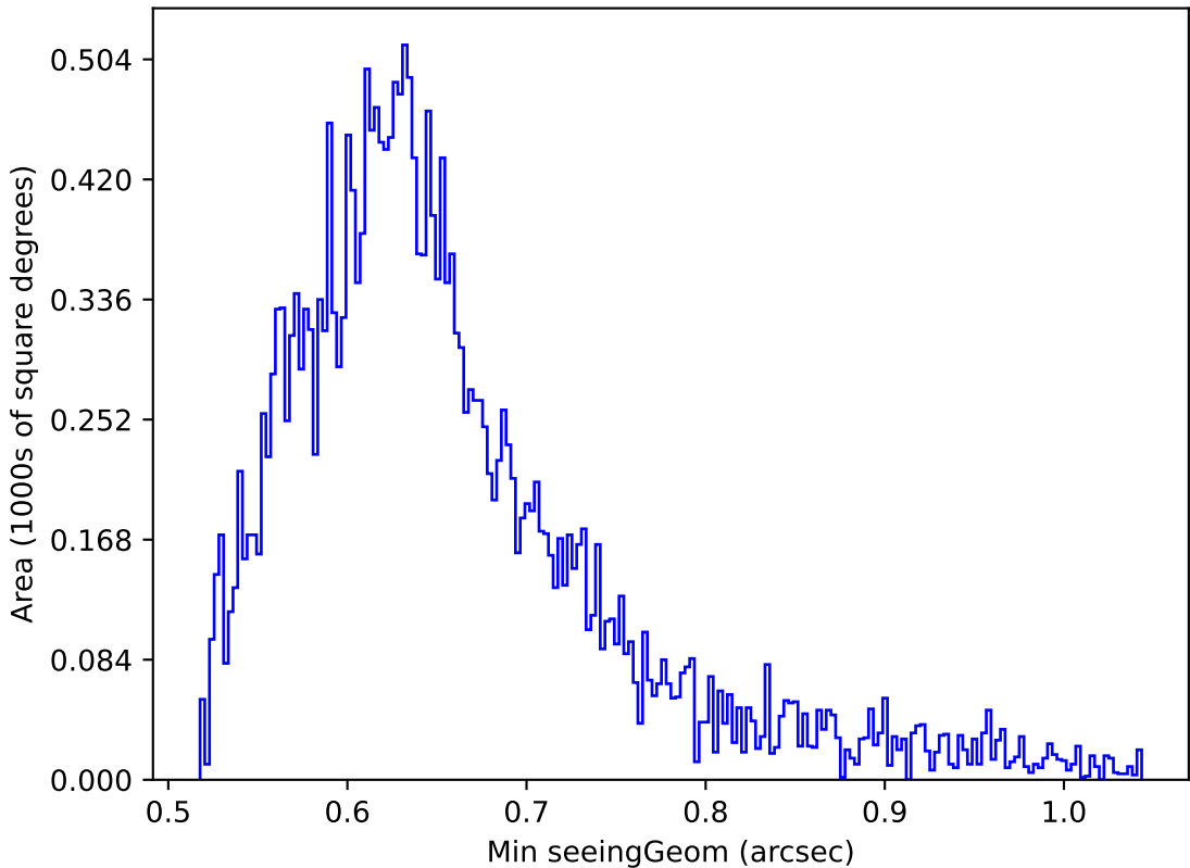
weather_cloudso36v3.4_10yrs Yr 1 z band: Min seeingGeom
