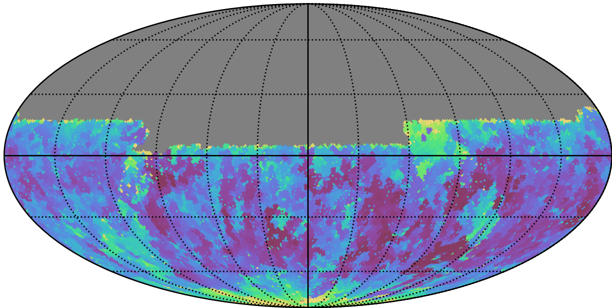
weather_cloudso36v3.4_10yrs Yr 1 y band: Min seeingGeom
