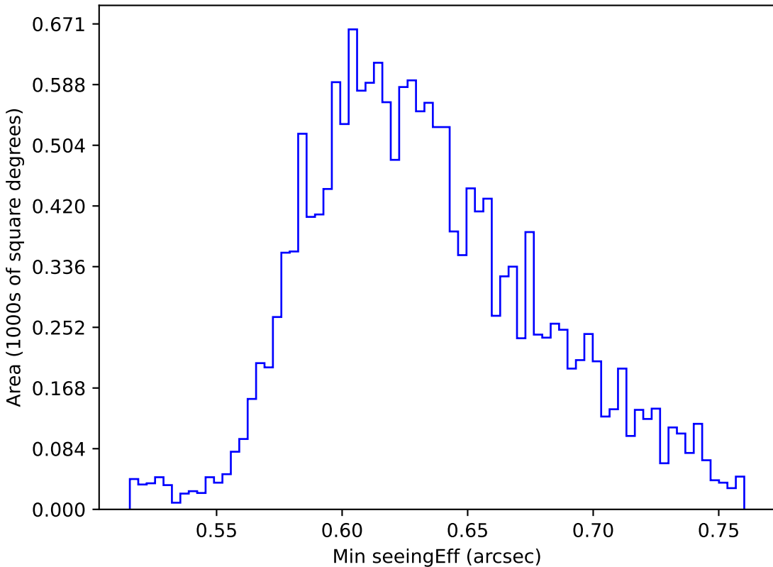
weather_cloudso36v3.4_10yrs WFD y band: Min seeingEff
