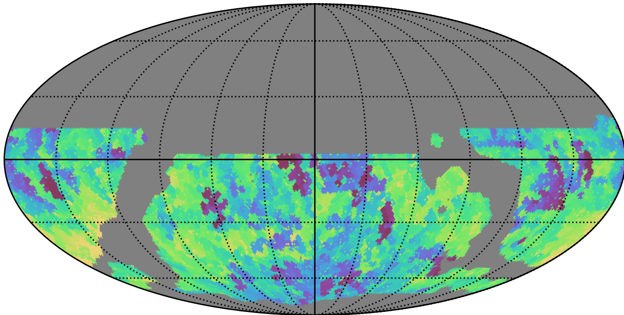
weather_cloudso36v3.4_10yrs WFD z band: Min saturation_mag
