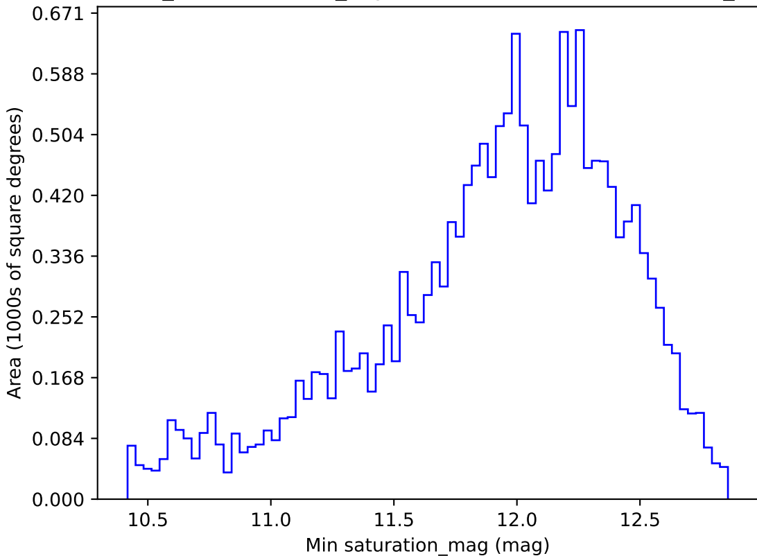
weather_cloudso36v3.4_10yrs WFD z band: Min saturation_mag
