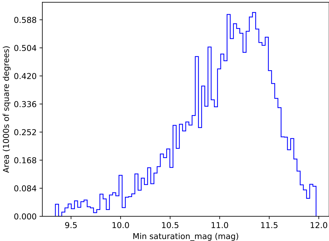
weather_cloudso36v3.4_10yrs WFD y band: Min saturation_mag
