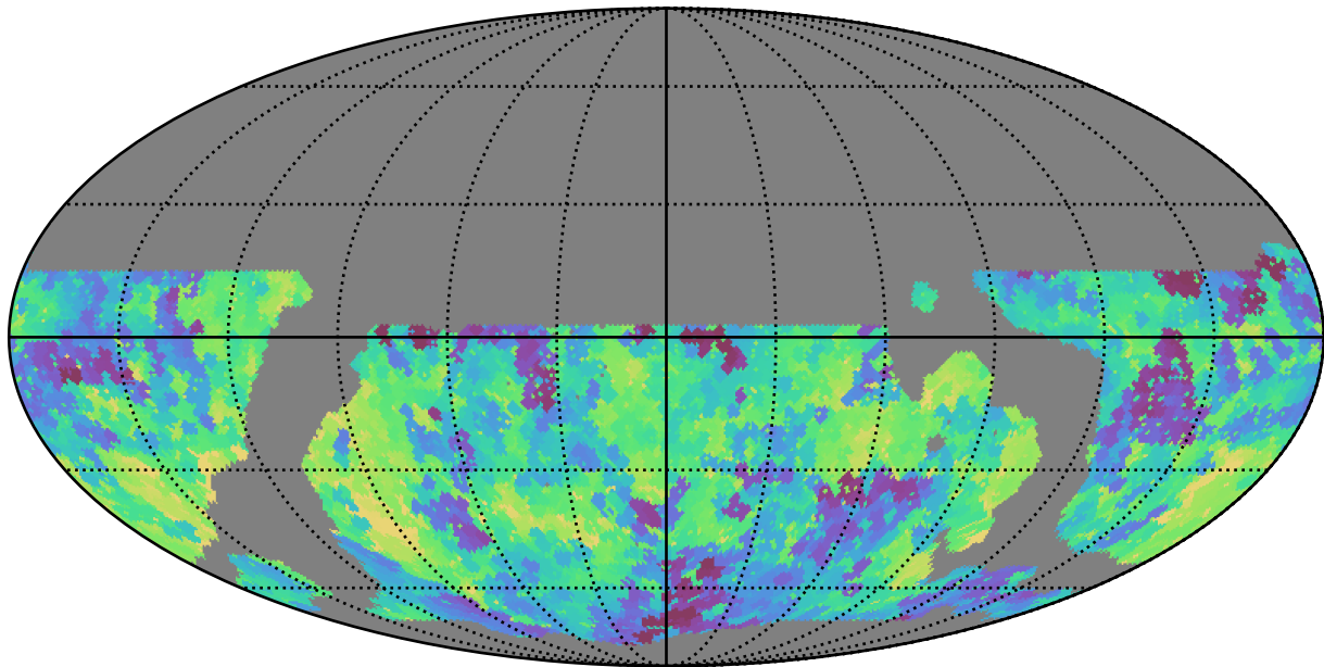
weather_cloudso36v3.4_10yrs WFD i band: Min saturation_mag
