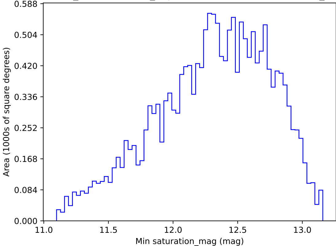
weather_cloudso36v3.4_10yrs WFD i band: Min saturation_mag
