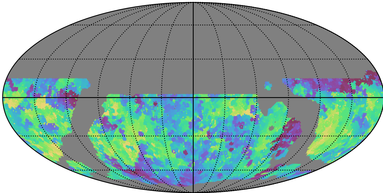
weather_cloudso36v3.4_10yrs WFD g band: Min saturation_mag
