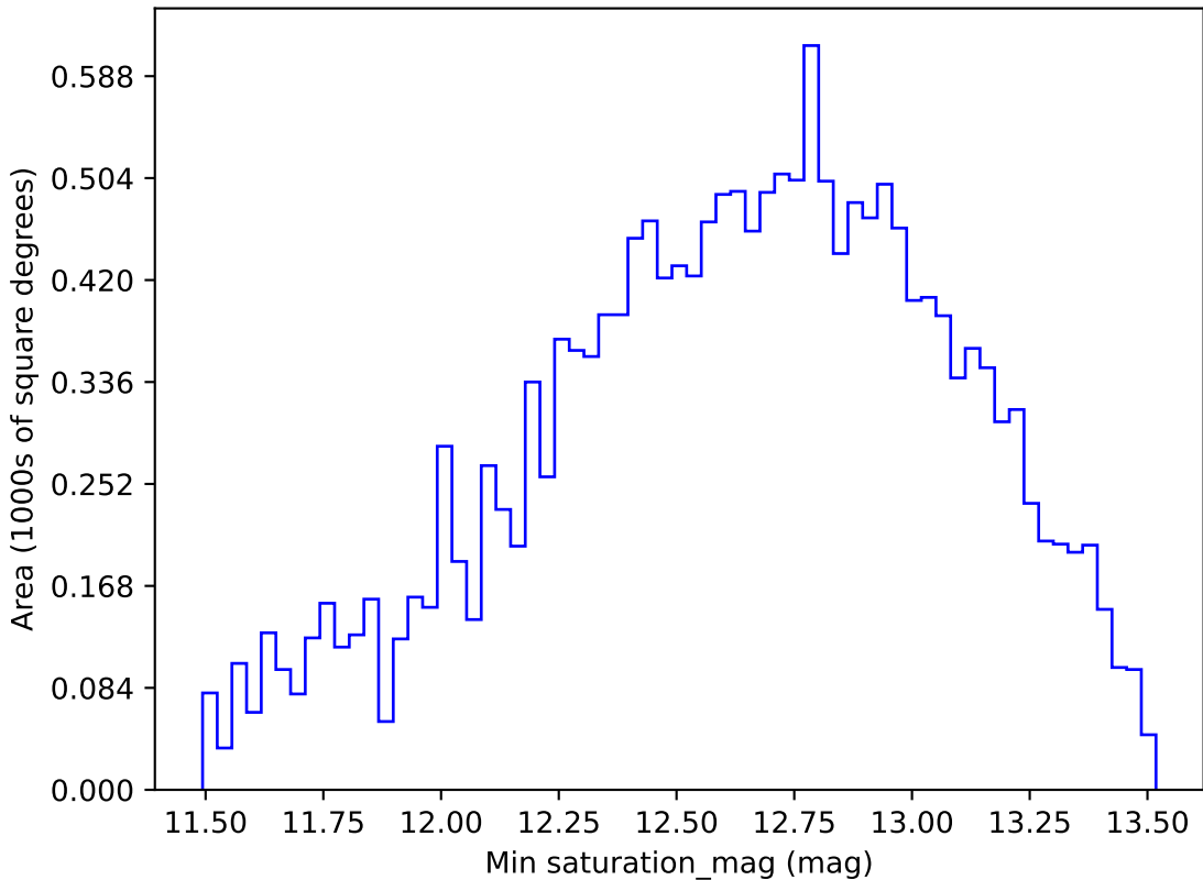
weather_cloudso36v3.4_10yrs WFD g band: Min saturation_mag
