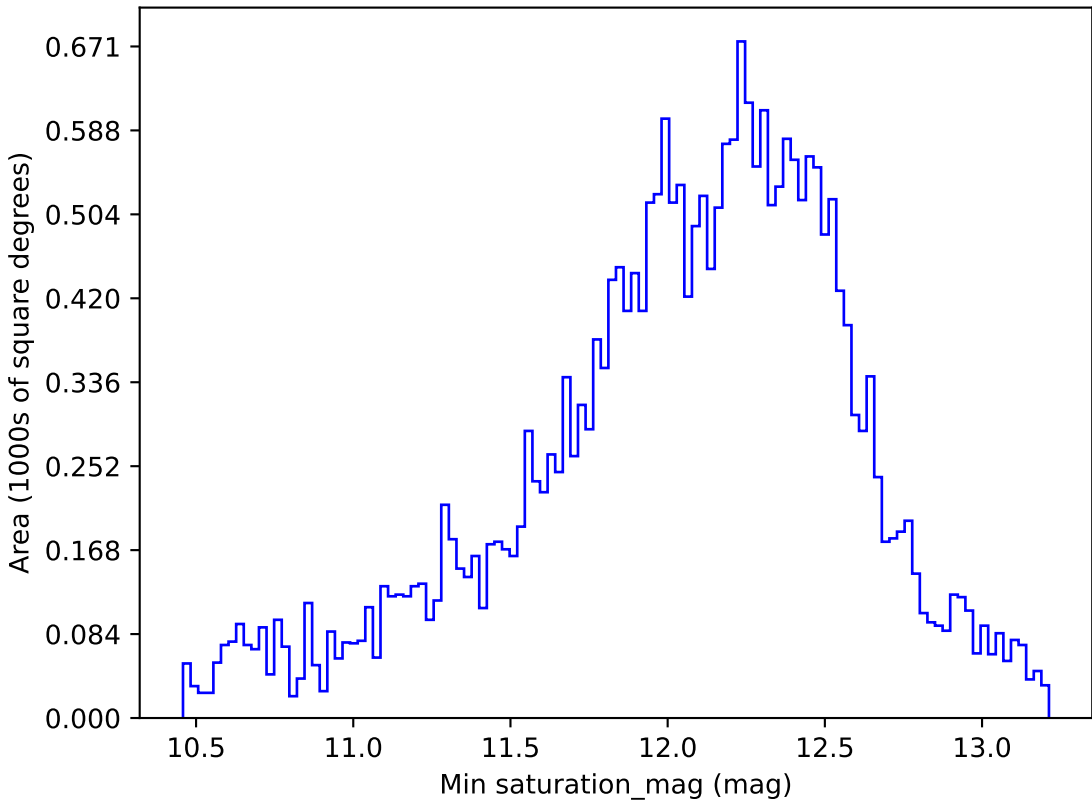
weather_cloudso36v3.4_10yrs All sky z band: Min saturation_mag
