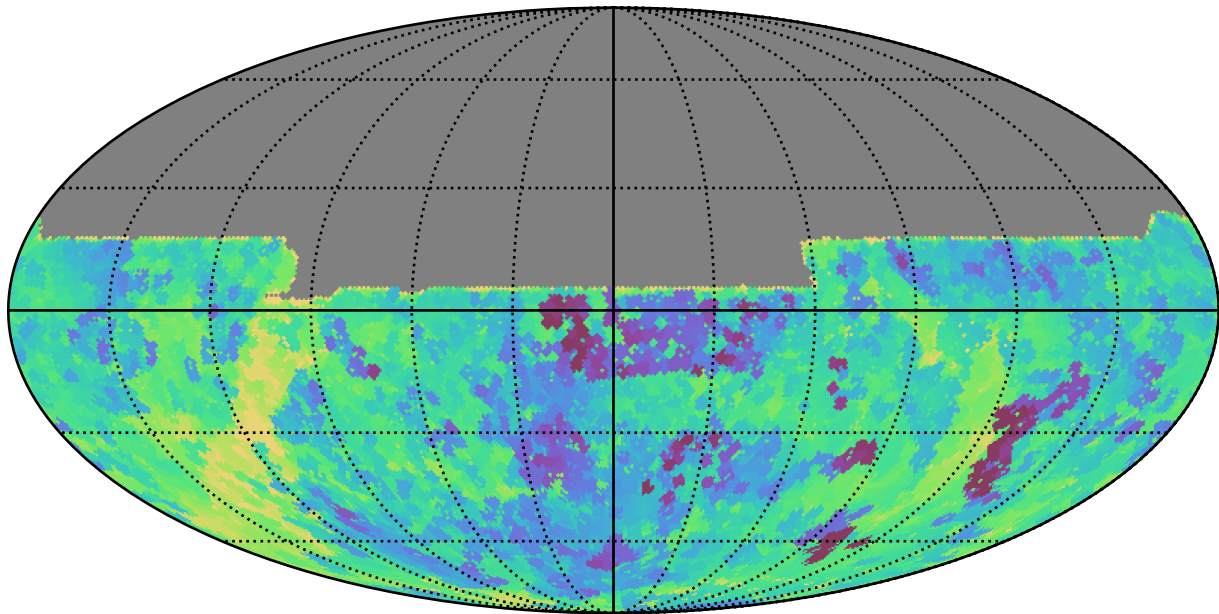
weather_cloudso36v3.4_10yrs All sky y band: Min saturation_mag
