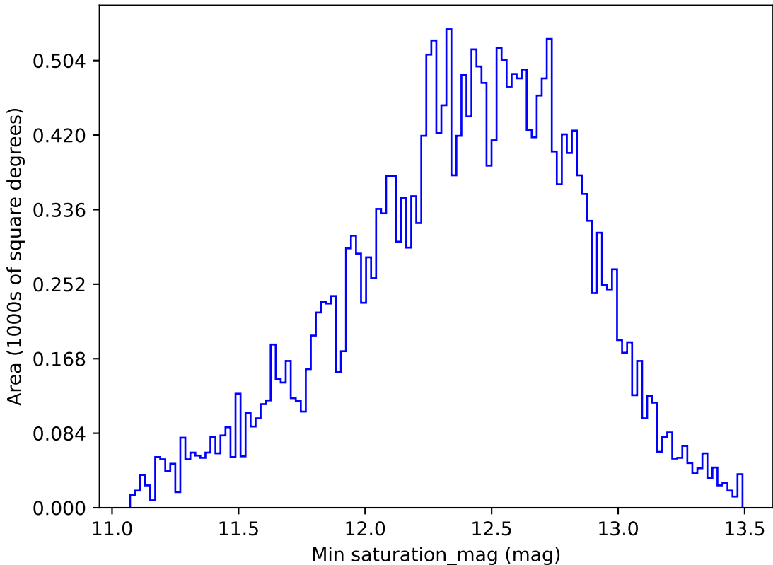
weather_cloudso36v3.4_10yrs All sky i band: Min saturation_mag
