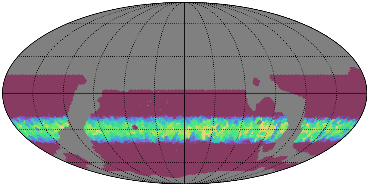
weather_cloudso36v3.4_10yrs WFD z band: Min normairmass
