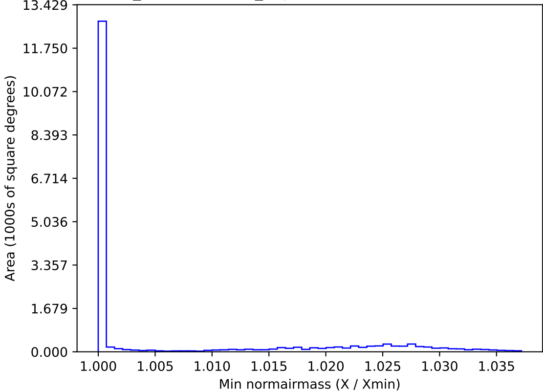
weather_cloudso36v3.4_10yrs WFD z band: Min normairmass
