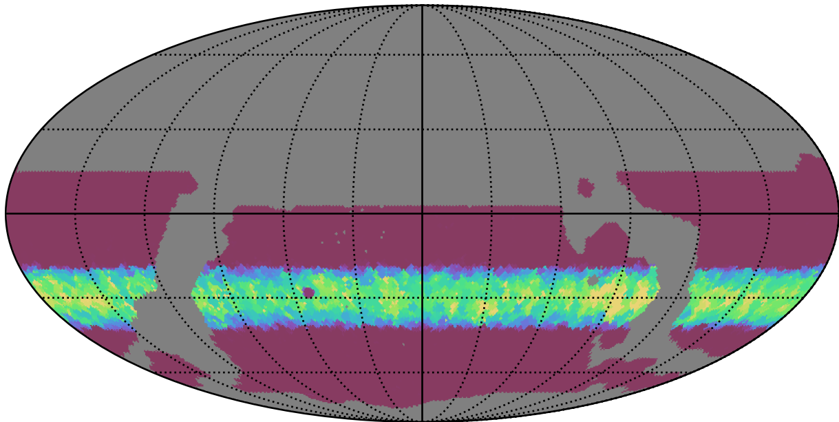
weather_cloudso36v3.4_10yrs WFD y band: Min normairmass
