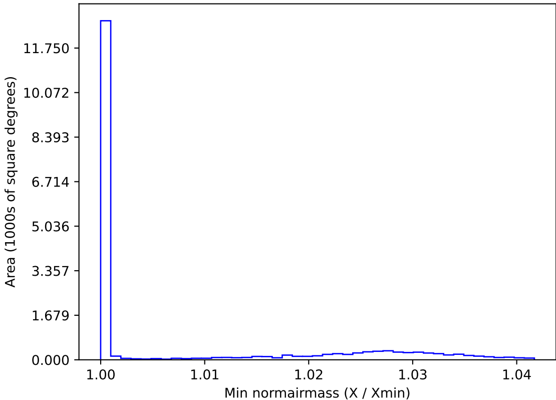
weather_cloudso36v3.4_10yrs WFD y band: Min normairmass
