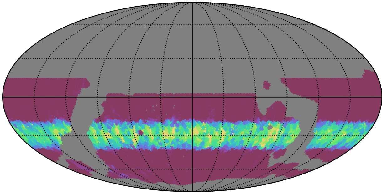
weather_cloudso36v3.4_10yrs WFD u band: Min normairmass
