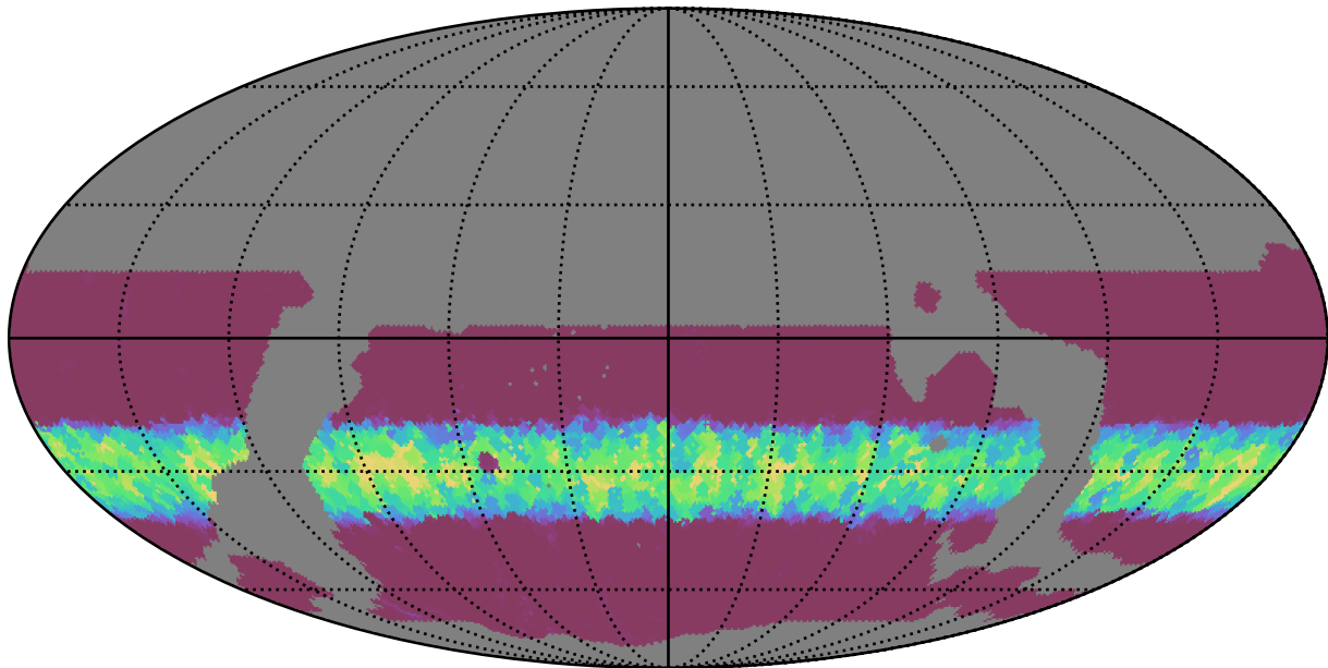
weather_cloudso36v3.4_10yrs WFD g band: Min normairmass
