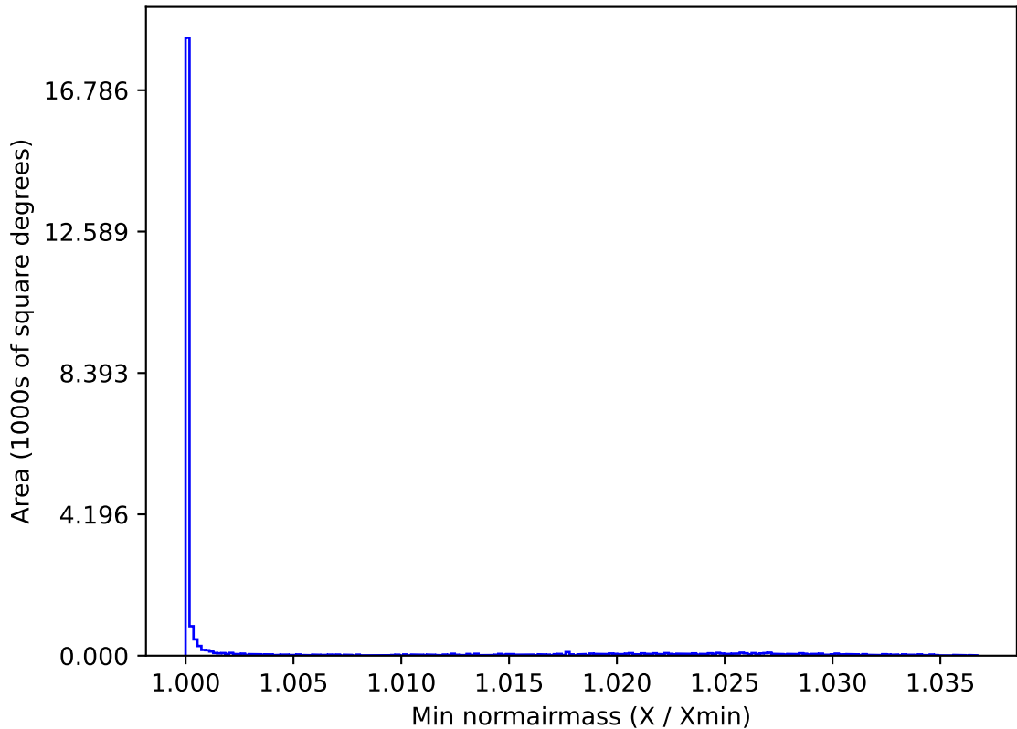
weather_cloudso36v3.4_10yrs All sky r band: Min normairmass
