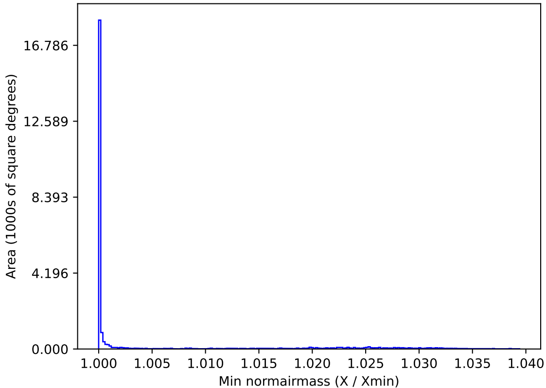
weather_cloudso36v3.4_10yrs All sky i band: Min normairmass
