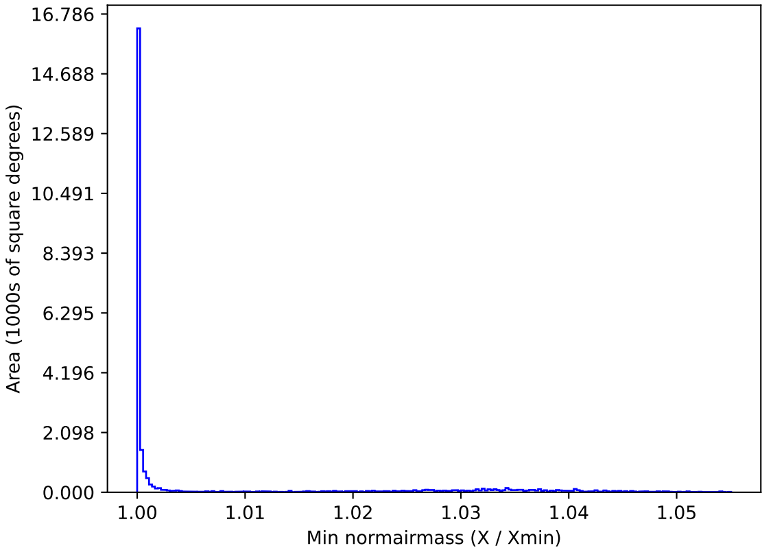
weather_cloudso36v3.4_10yrs All sky g band: Min normairmass
