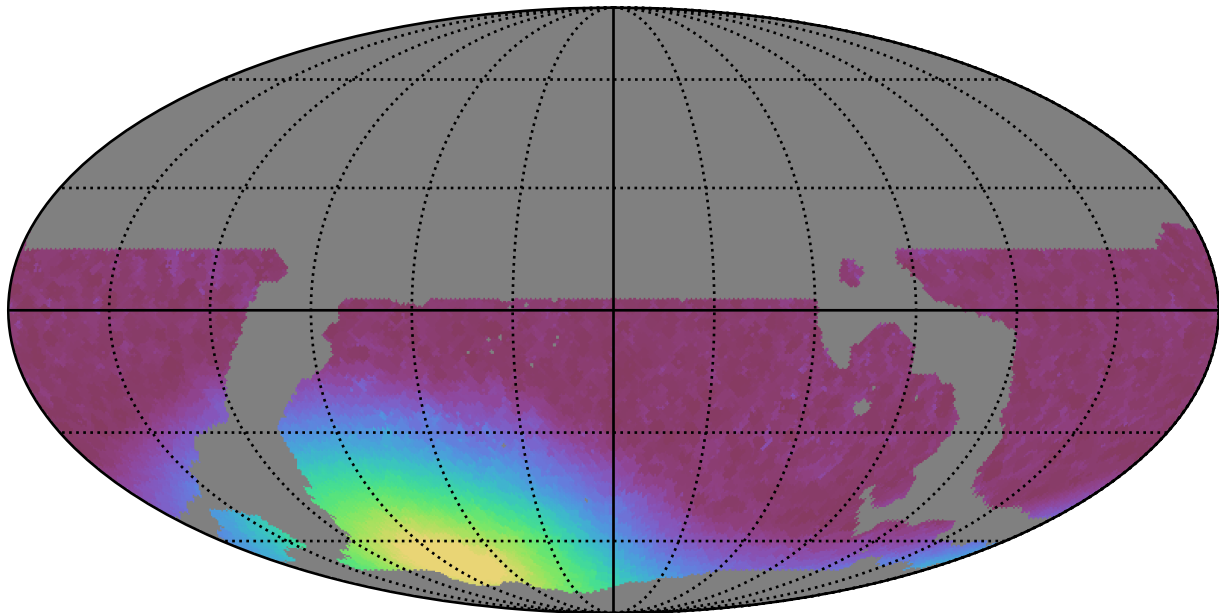
weather_cloudso36v3.4_10yrs WFD i band: Min moonDistance
