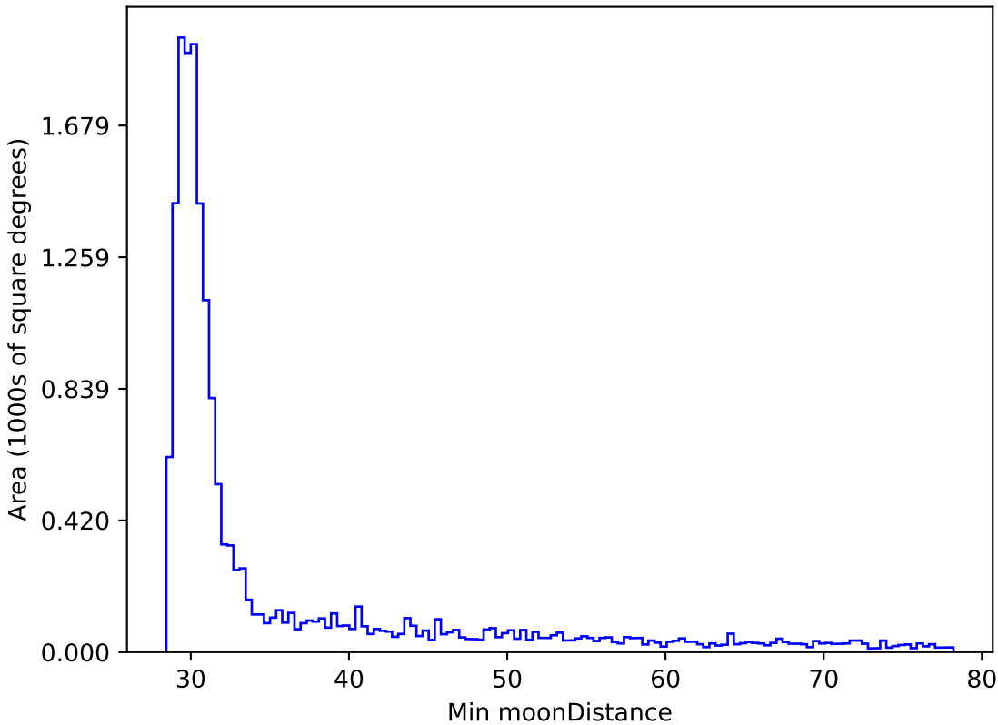
weather_cloudso36v3.4_10yrs WFD i band: Min moonDistance
