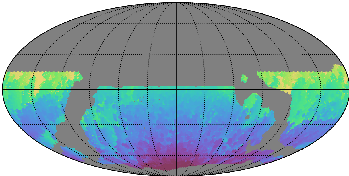
weather_cloudso36v3.4_10yrs WFD z band: Min HA
