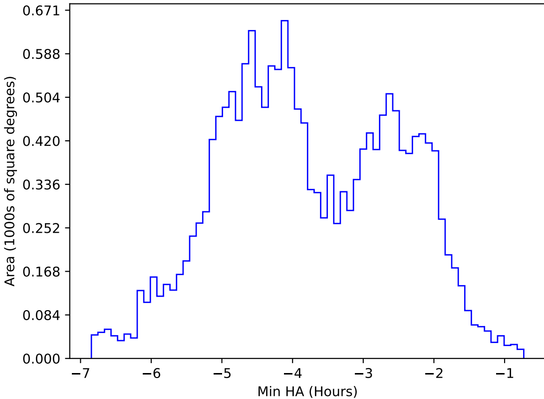
weather_cloudso36v3.4_10yrs WFD y band: Min HA
