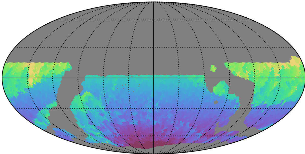
weather_cloudso36v3.4_10yrs WFD r band: Min HA
