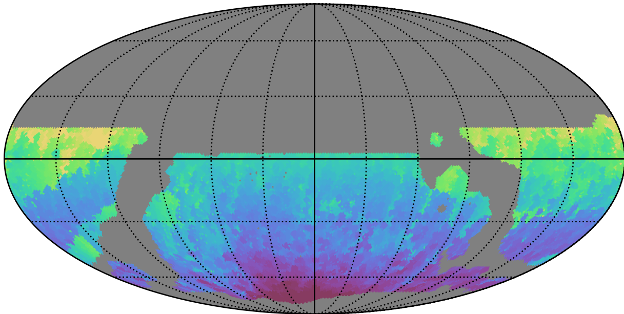
weather_cloudso36v3.4_10yrs WFD i band: Min HA
