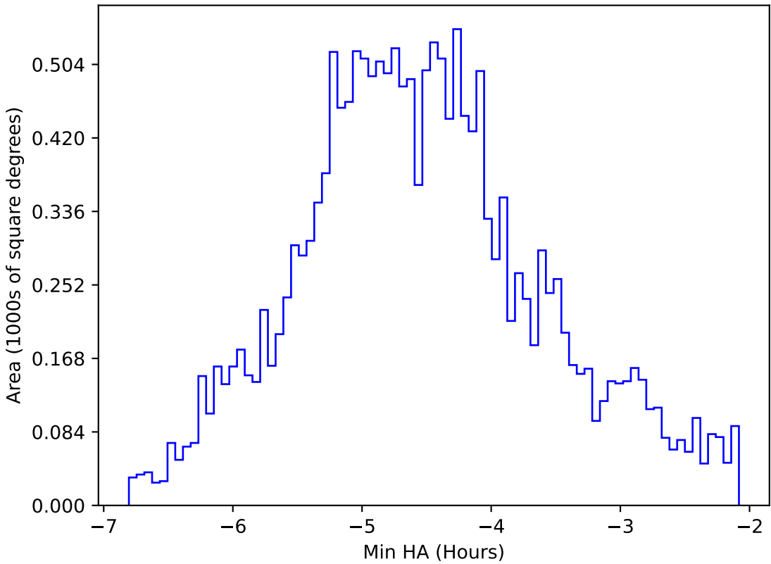
weather_cloudso36v3.4_10yrs WFD i band: Min HA
