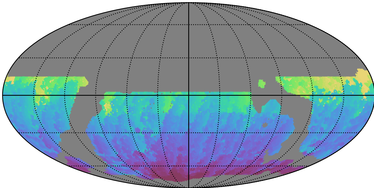
weather_cloudso36v3.4_10yrs WFD g band: Min HA
