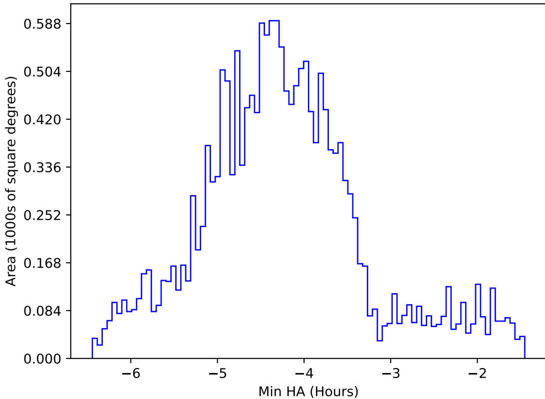
weather_cloudso36v3.4_10yrs WFD g band: Min HA
