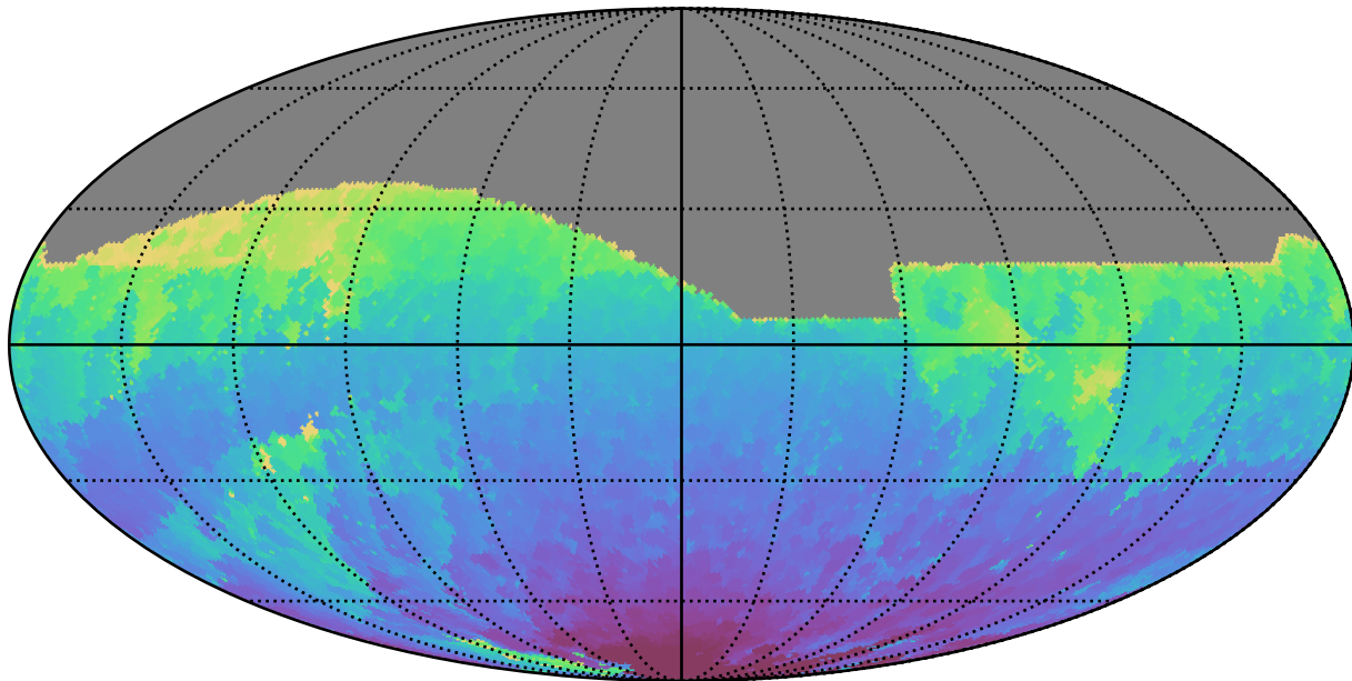
weather_cloudso36v3.4_10yrs All sky z band: Min HA
