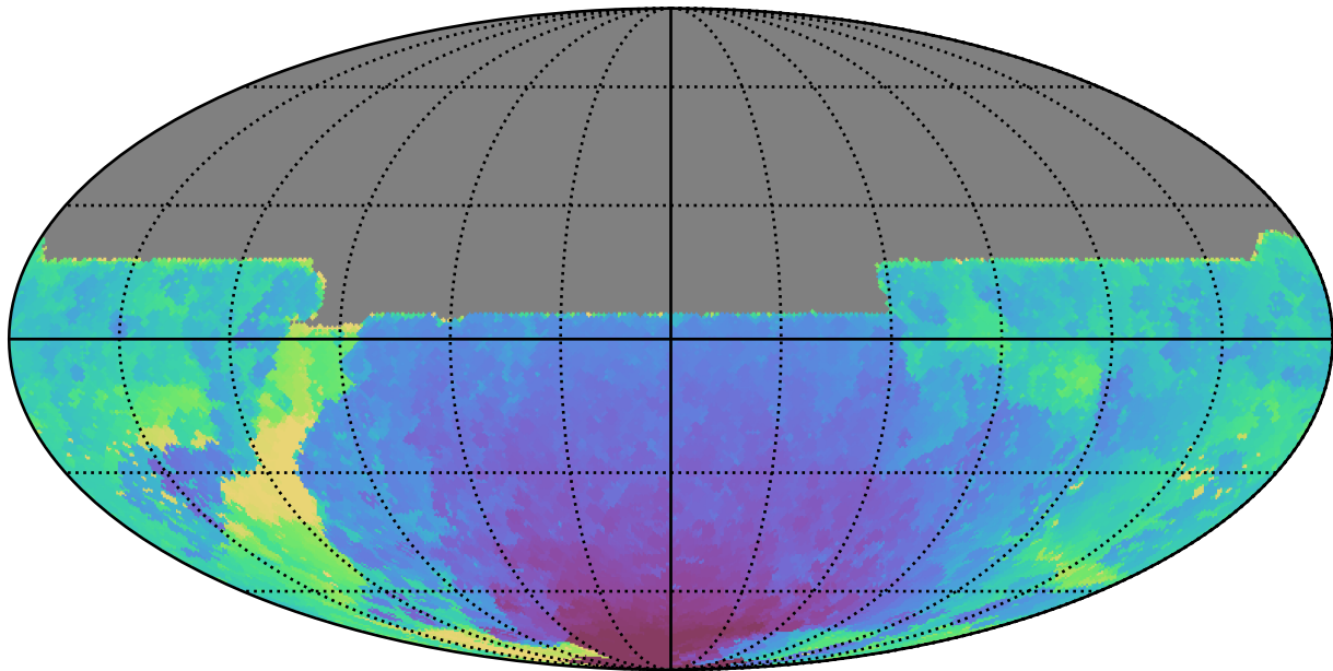
weather_cloudso36v3.4_10yrs All sky y band: Min HA
