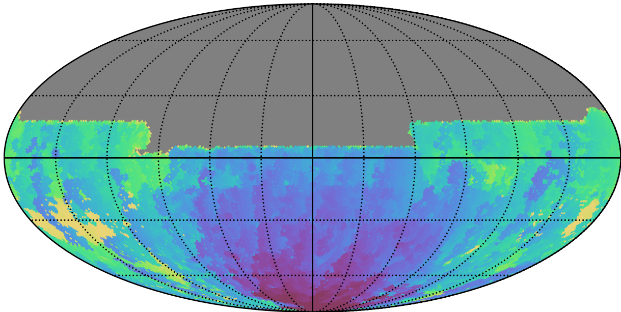
weather_cloudso36v3.4_10yrs All sky u band: Min HA
