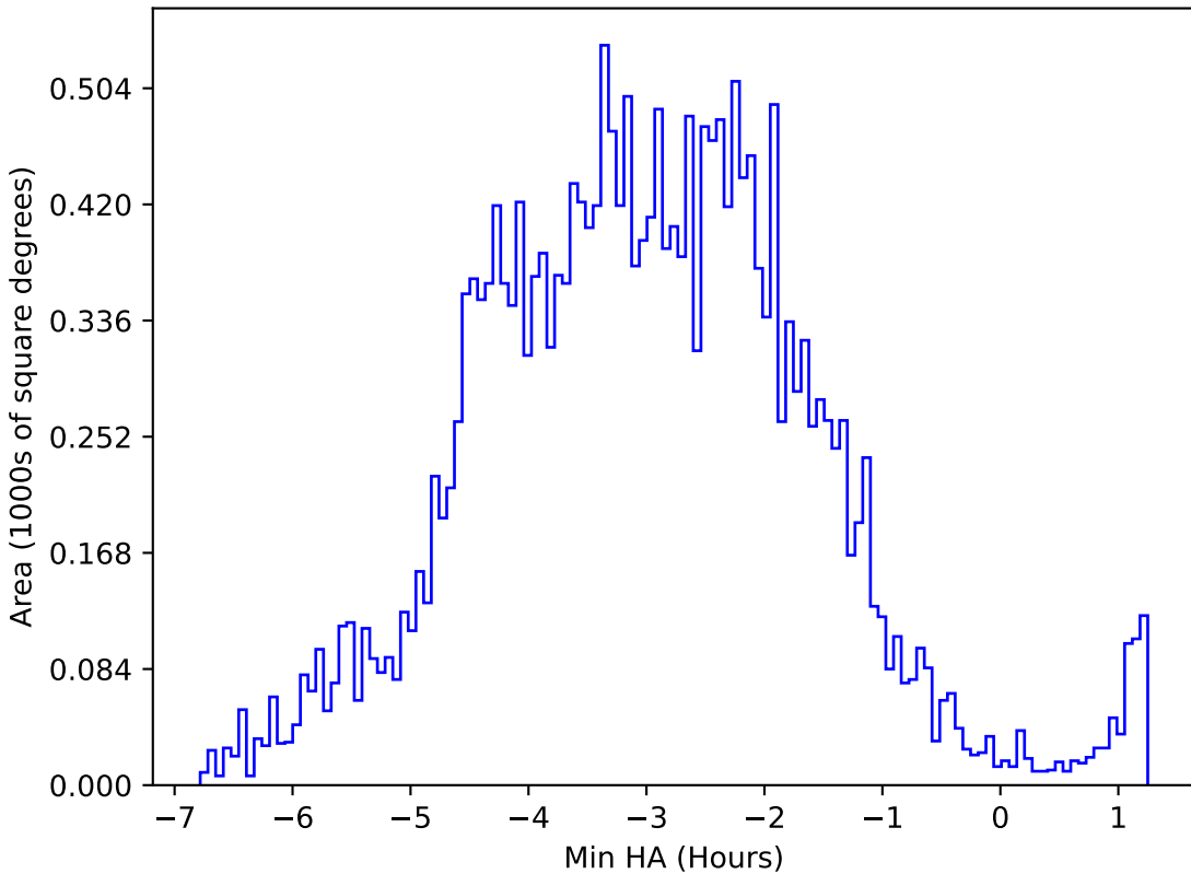
weather_cloudso36v3.4_10yrs All sky u band: Min HA
