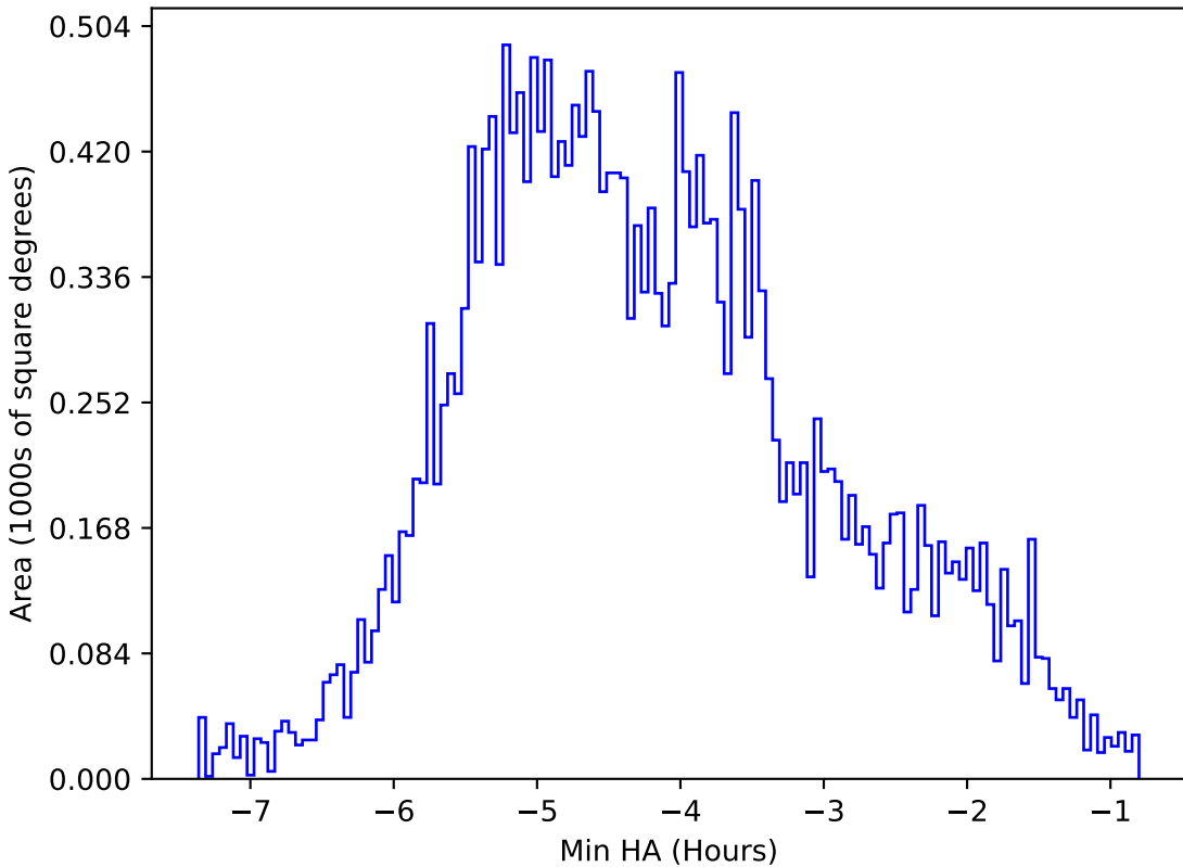
weather_cloudso36v3.4_10yrs All sky r band: Min HA
