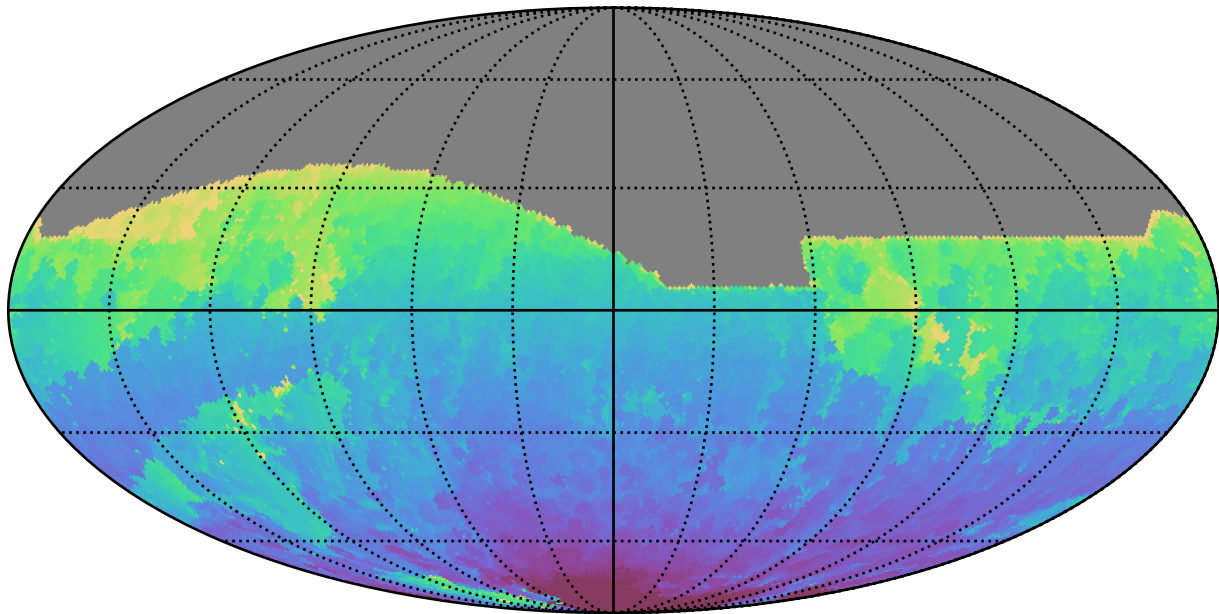
weather_cloudso36v3.4_10yrs All sky i band: Min HA
