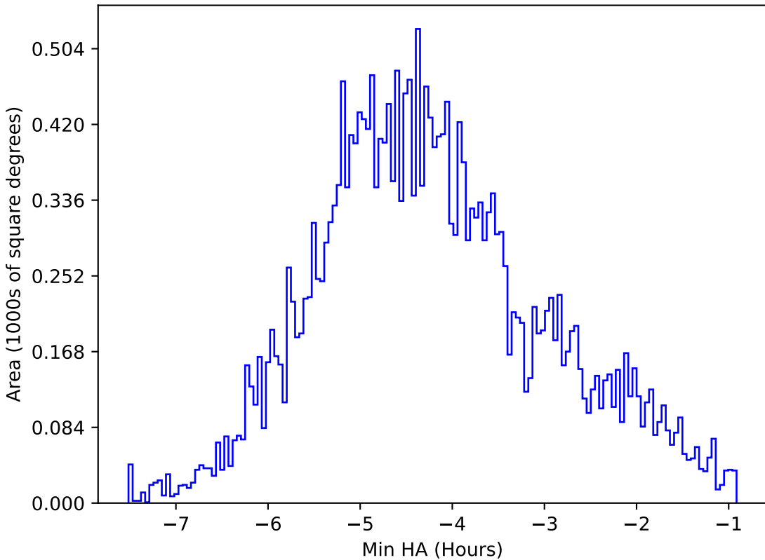
weather_cloudso36v3.4_10yrs All sky i band: Min HA
