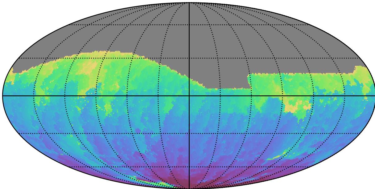
weather_cloudso36v3.4_10yrs All sky g band: Min HA
