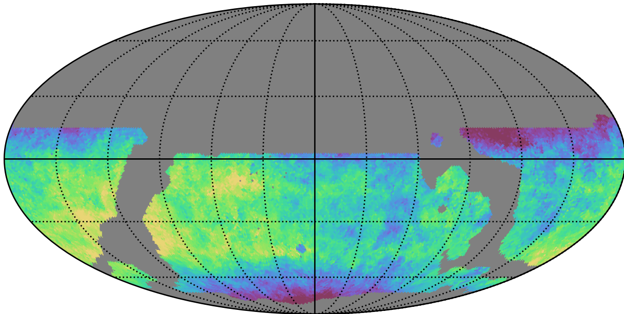
weather_cloudso36v3.4_10yrs WFD y band: Median saturation_mag
