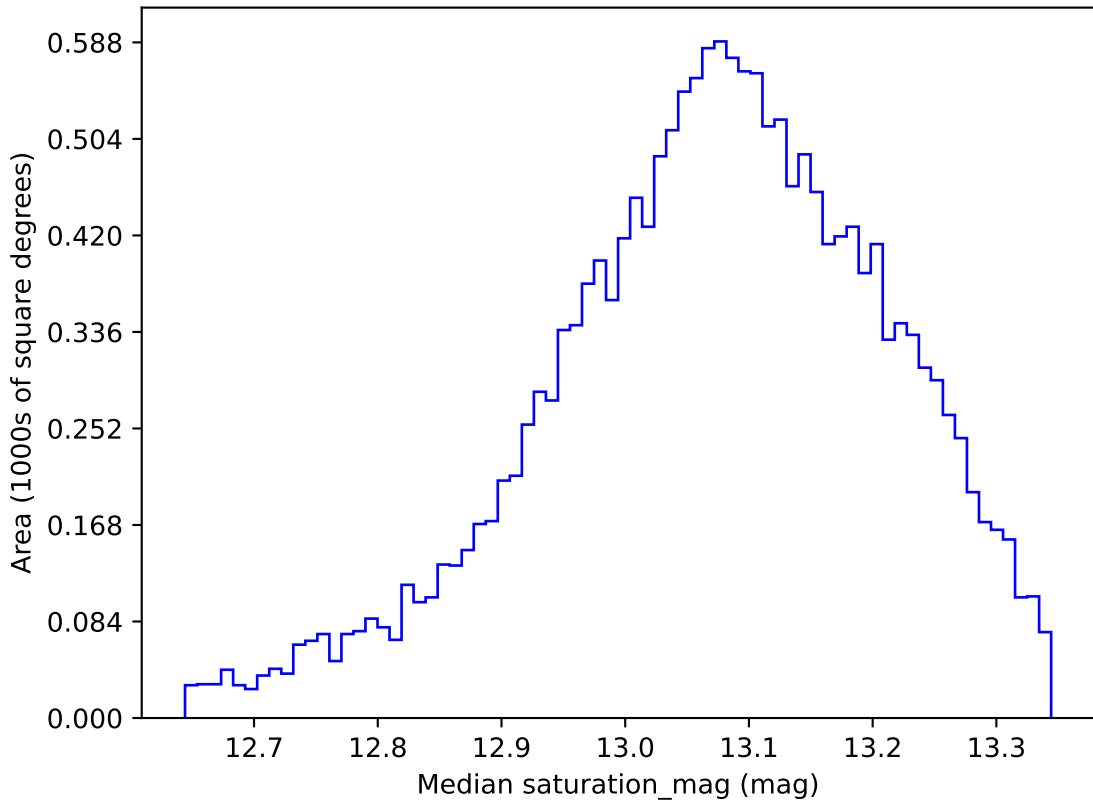
weather_cloudso36v3.4_10yrs WFD y band: Median saturation_mag
