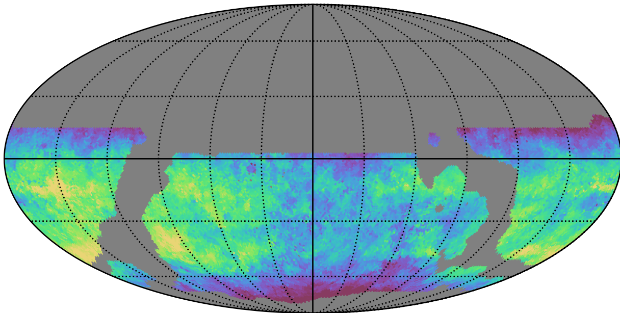
weather_cloudso36v3.4_10yrs WFD g band: Median saturation_mag
