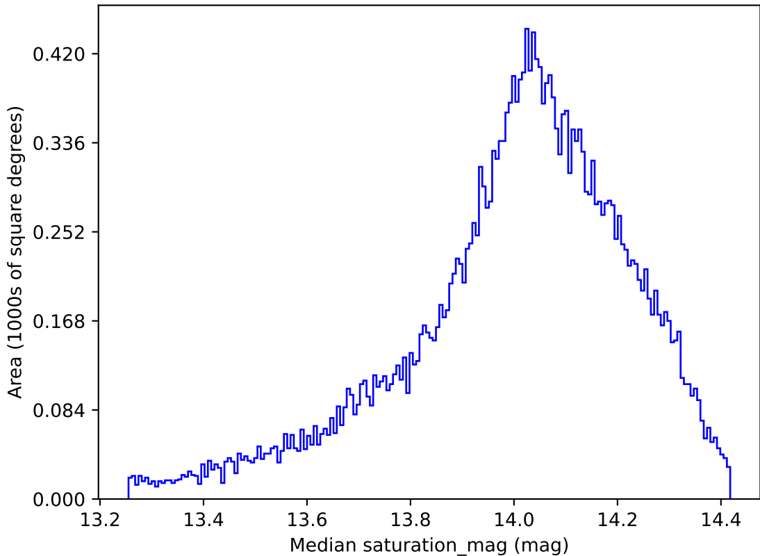
weather_cloudso36v3.4_10yrs All sky z band: Median saturation_mag
