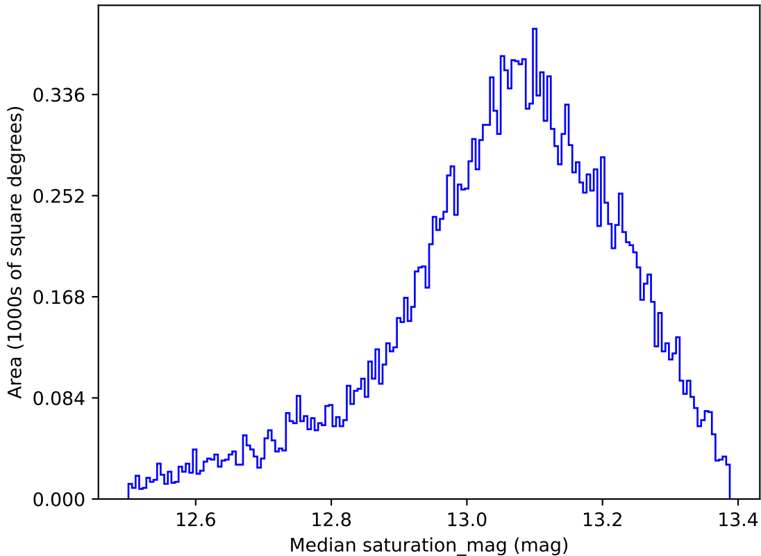
weather_cloudso36v3.4_10yrs All sky y band: Median saturation_mag
