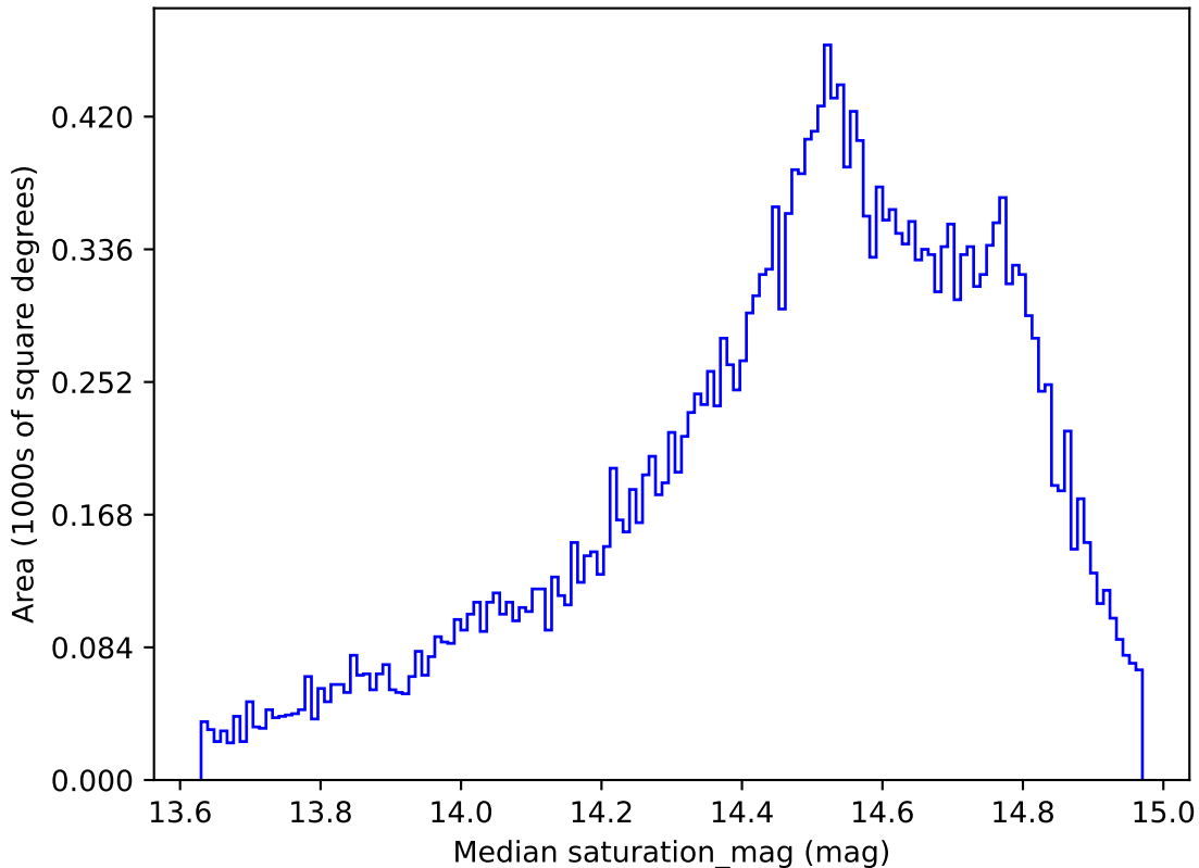
weather_cloudso36v3.4_10yrs All sky r band: Median saturation_mag
