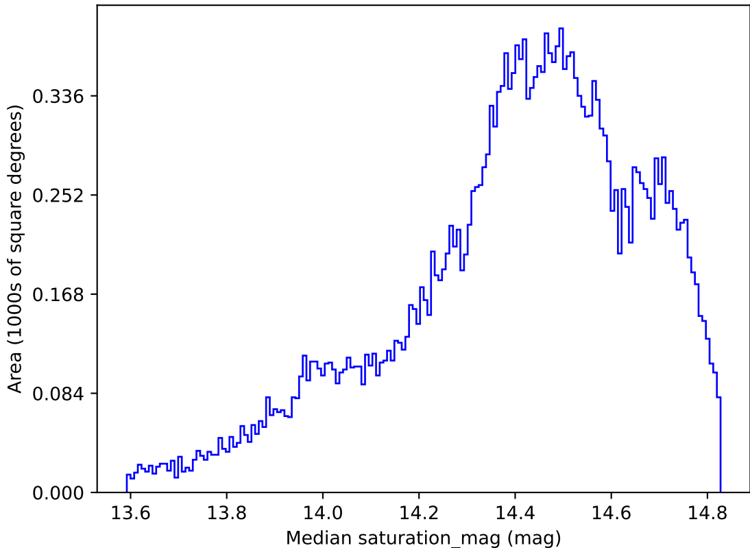
weather_cloudso36v3.4_10yrs All sky i band: Median saturation_mag
