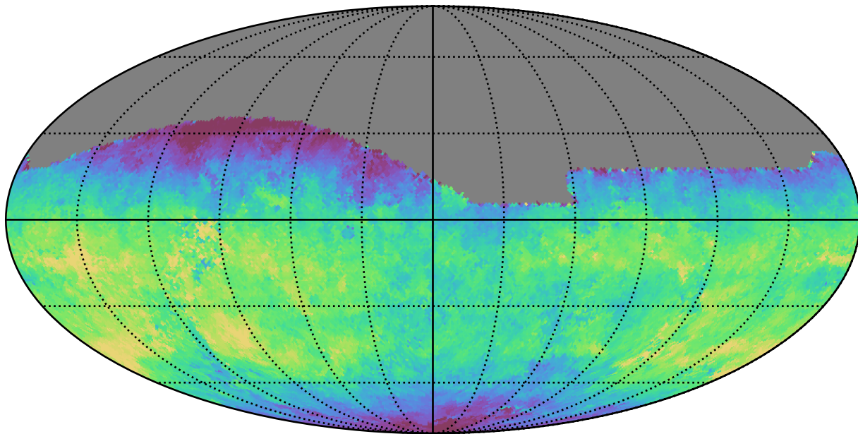
weather_cloudso36v3.4_10yrs All sky g band: Median saturation_mag
