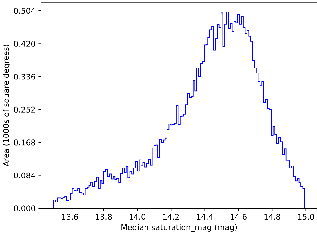
weather_cloudso36v3.4_10yrs All sky g band: Median saturation_mag
