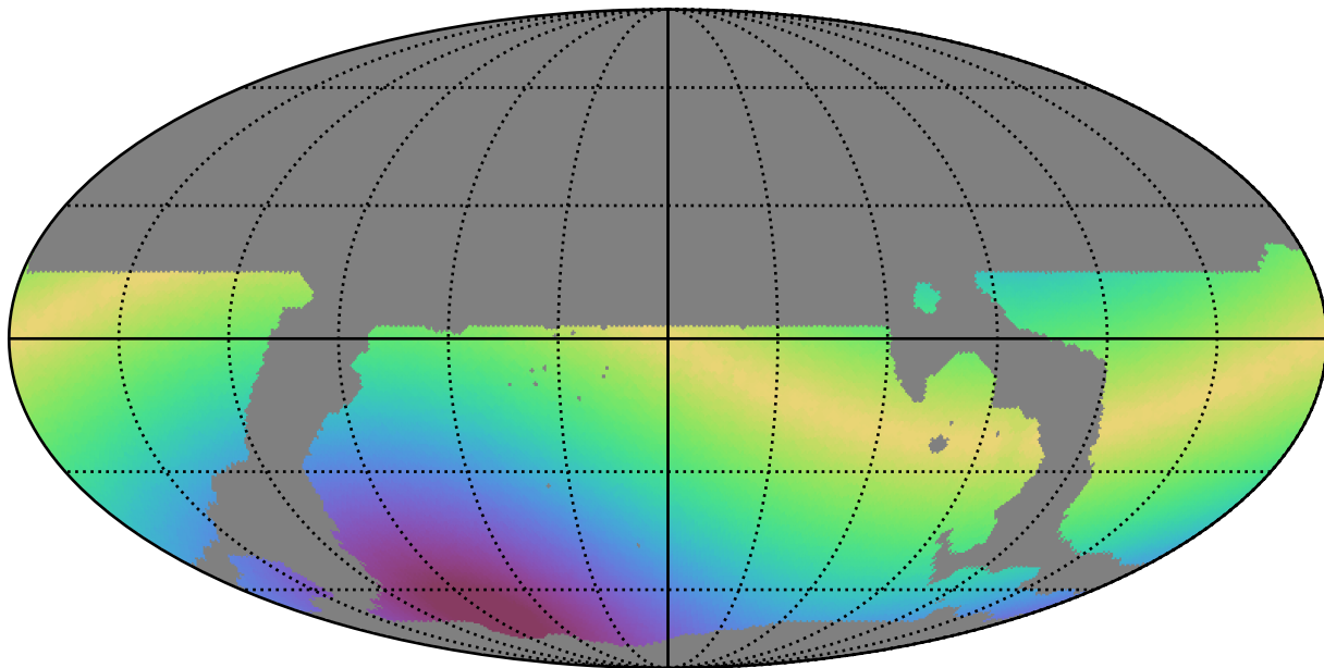
weather_cloudso36v3.4_10yrs WFD z band: Max solarElong
